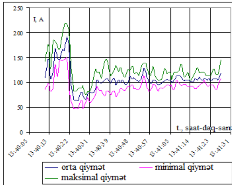
Şəkil 3. Ortalama müddəti 1 saniyə olduqda “Sənaye qovşağı” 220/110/10 kV yarımstansiyası tərəfdə Bakı Poladərilmə Şirkətinin 110 kV fazasında cərəyanın dəyişmə qrafiki
