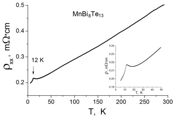
Рис. 4. Температурная зависимость удельного сопротивления \rho_{xx}(T) монокристаллов \text{MnBi}_8\text{Te}_{13} в интервале температур 5-300K. На вставке зависимость \rho_{xx}(T) в интервале температур 5-50K.
