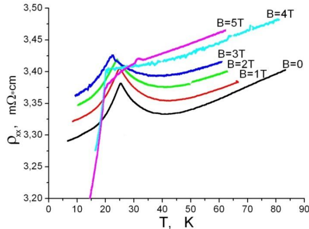
Рис. 2. Температурная зависимость удельного сопротивления \rho_{xx}(T) монокристаллов \text{MnBi}_2\text{Te}_4 во внешних магнитных полях B=0, 1, 2, 3, 4, 5 Т.
