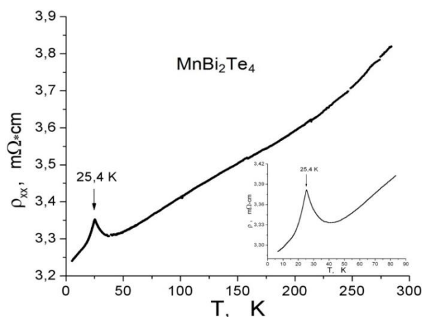
Рис. 1. Температурная зависимость удельного сопротивления \rho_{xx}(T) монокристаллов \text{MnBi}_2\text{Te}_4 в интервале температур 5-300K. На вставке зависимость \rho_{xx}(T) в интервале температур 5-90K.
