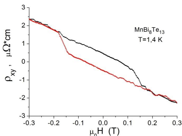
Рис. 6. Магнитопольевая зависимость холловского сопротивления \rho_{xy}(B) при температуре T = 1,4 \text{ K} .
