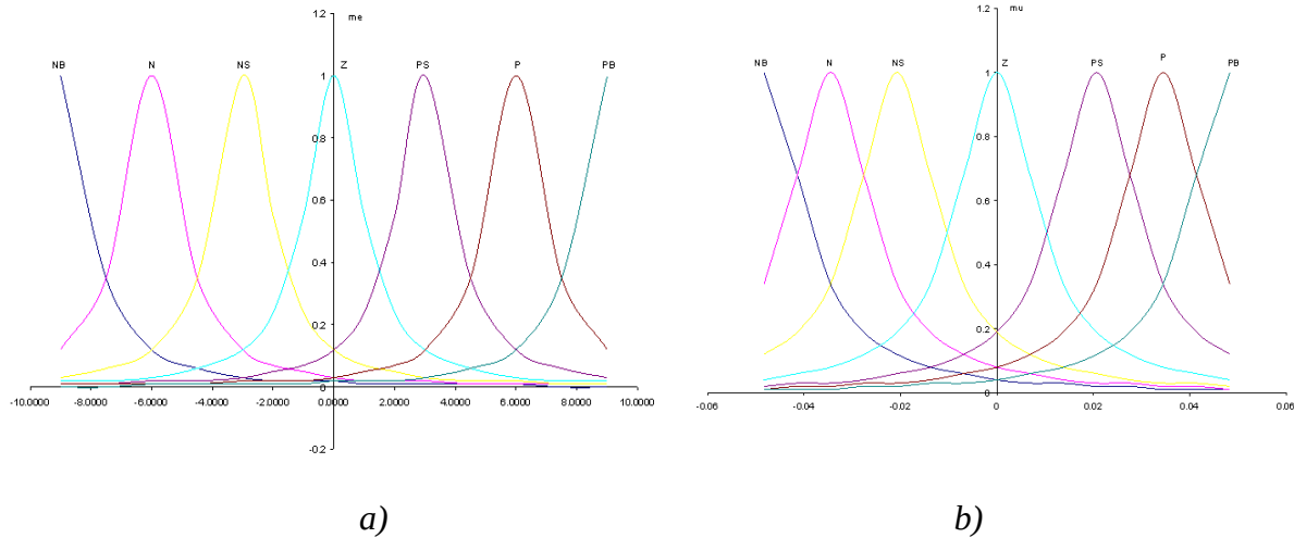
Şəkil 1. Buxar generatorunun: a) temperaturunun idarəedilməsinin xətasının termlərinin (qeyri-səlis çoxluqlarının) mənsubiyyət funksiyaları; b) idarəedici təsirin termlərinin (qeyri-səlis çoxluqlarının) mənsubiyyət funksiyaları.
