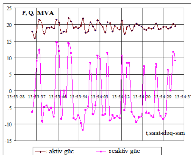
Şəkil 1. “Bakı Poladəritmə şirkəti” MMC-nin 110 kV-luq 2 sayılı hava xəttinin “Sənaye qovşağı” yarımstansiyasından aktiv və reaktiv gücünün qeydiyyatının nəticələri
