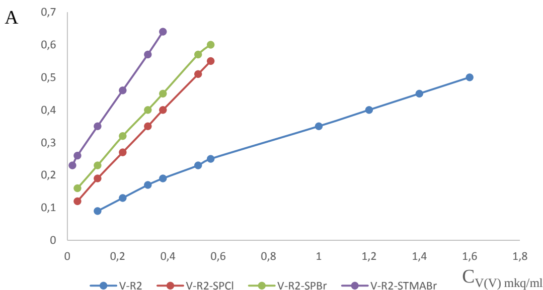
Şəkil 2. Vanadiumun (V) ionunun R2 reagenti ilə binar və müxtəlifliqandlı komplekslər şəklində təyininin dərəcəli qrafiki. \lambda_{max} = 490 \text{ nm} , C_{metal} = 10^{-2} \text{ mg/ml}
