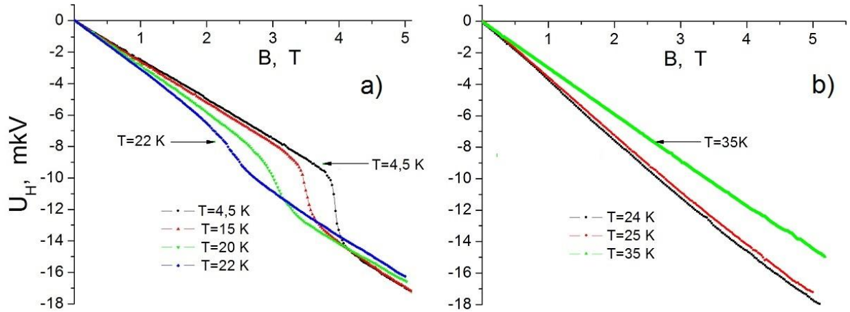
Рис. 3. Магнитополевая зависимость холловского напряжения U_H(B) при температурах а) T = 4,5; 15; 20; 22\text{ K} и б) T = 24; 25 и 35\text{ K} .
