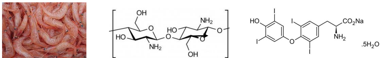
Şəkil 1. Xitozanın təbii mənbəsi və kimyəvi strukturu, LTH-Na molekulu
